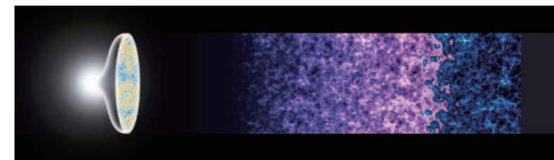
宇宙が誕生後38万年で一度中性化したのち、その後誕生する初代星や銀河によって再電離していく様子。
