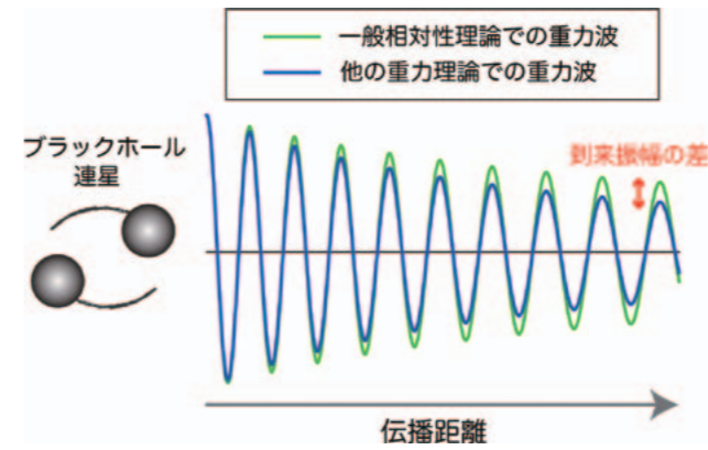
重力波の観測を用いた重力理論検証の概念図。2016年に幕を開けた重力波天文学は今後大きな進展が期待できる分野である。
