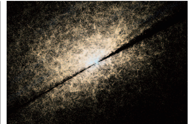
SDSSにより明らかになった宇宙の大規模な構造。
