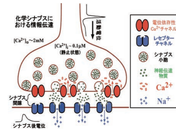
Fig.2 化学シナプスにおける情報伝達
