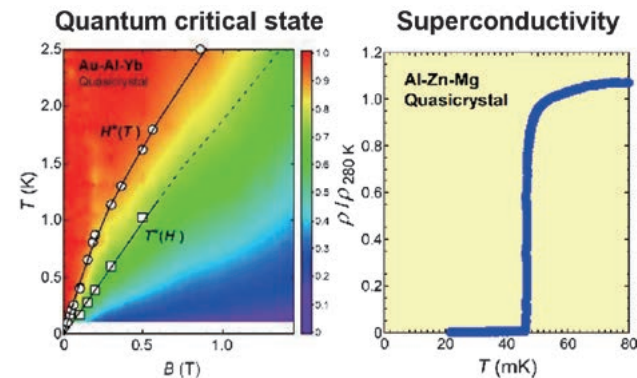
図4：Au-Al-Yb準結晶の量子臨界現象とAl-Zn-Mg準結晶の超伝導
