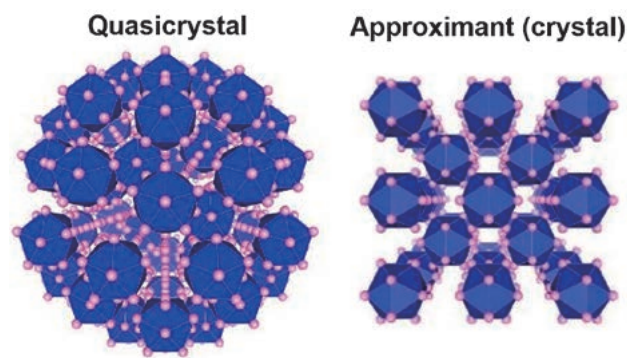
図3：Au-Al-Yb準結晶と近似結晶（結晶）の構造モデル
