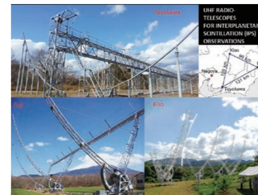
太陽風観測専用のUHF帯電波望遠鏡群
